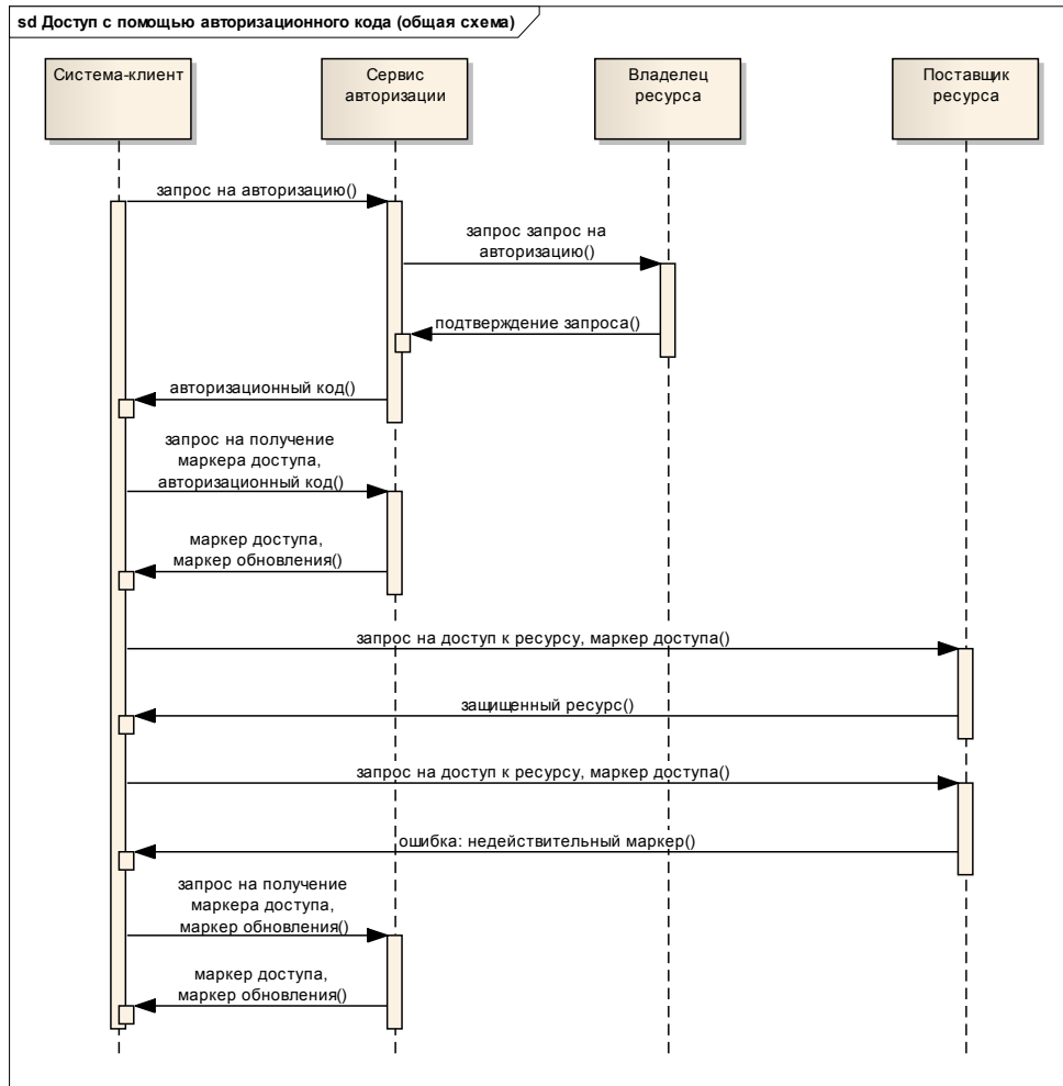
Рисунок 16 – Общая схема взаимодействия при получении маркера доступа с помощью авторизационного кода
