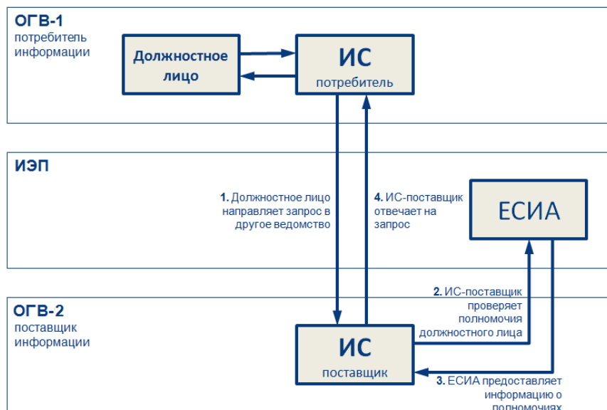
Рисунок 6 – Получение данных о полномочиях должностного лица
