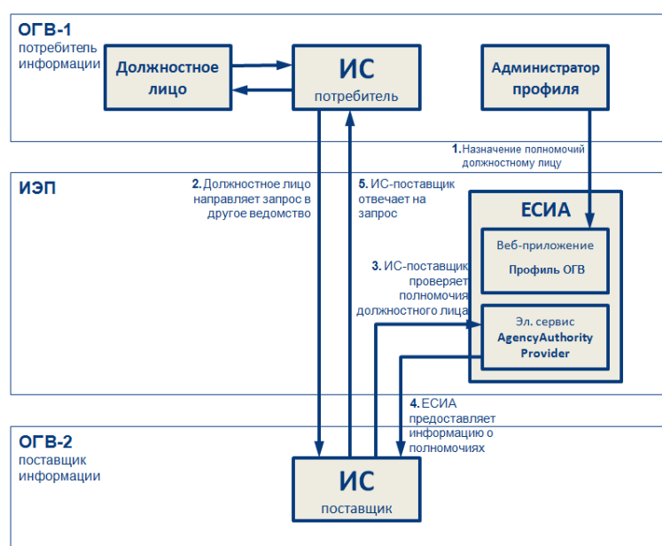
Рисунок 7 – Предоставление полномочий и авторизация должностных лиц
