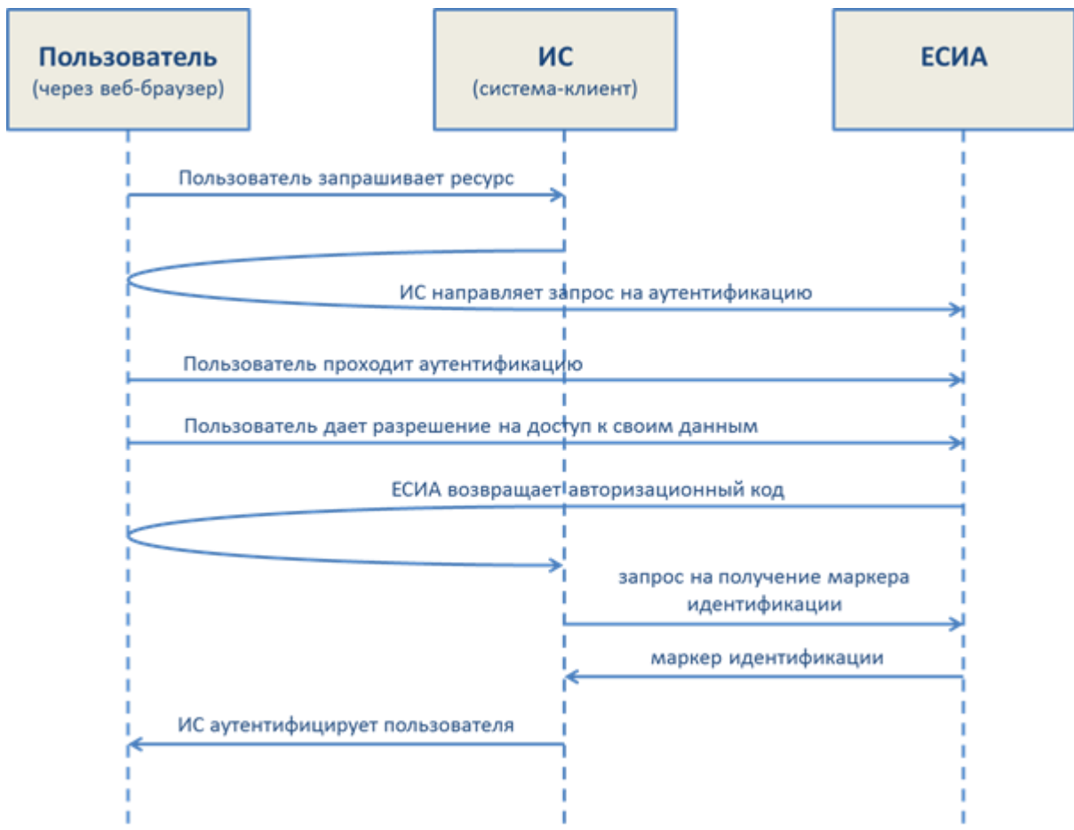
Рисунок 4 – Идентификация и аутентификация пользователей при использовании механизма OAuth 2.0
