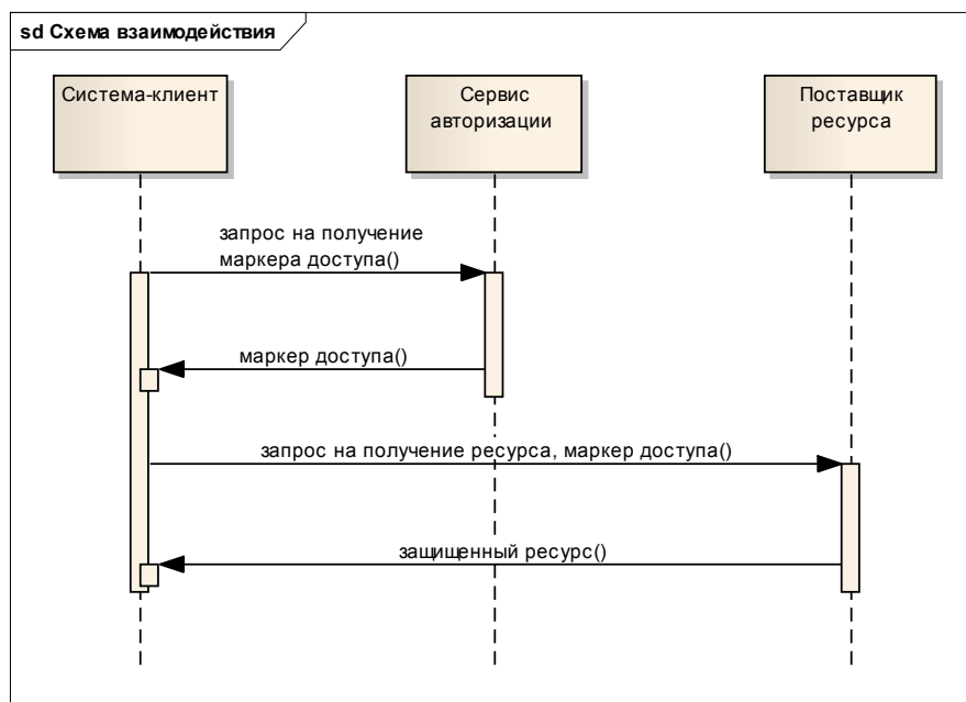
Рисунок 17 – Схема взаимодействия при реализации модели контроля доступа на основе полномочий системы-клиента
